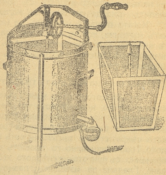
Фигура 4. Центрофуга за медъ,
